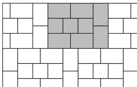
Vzor pokládky XL-p05
