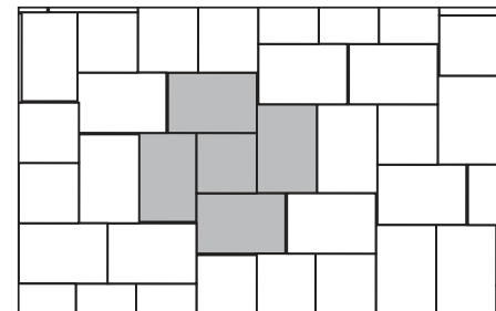
Vzor pokládky XL-p03
