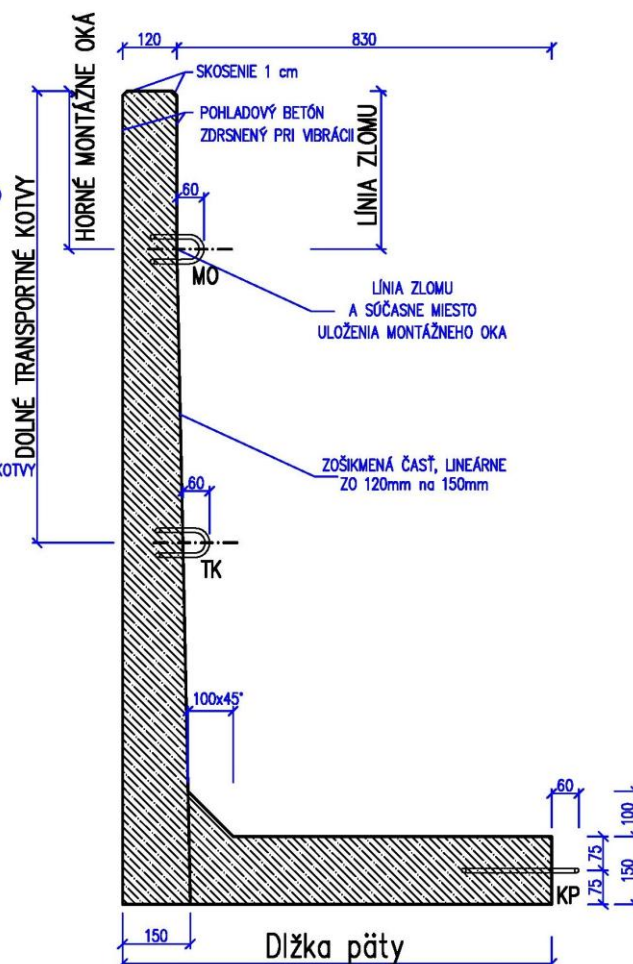
REZ A-A M=1:10
