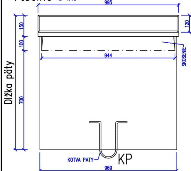
PODORYS M=1:10
