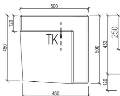
PODORYS M=1:10
