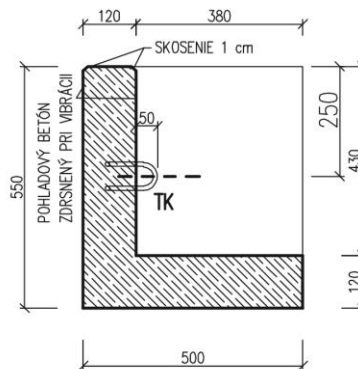
REZ A-A M=1:10
