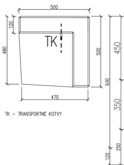
PODORYS M=1:10
