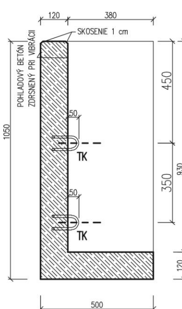
REZ A-A M=1:10
