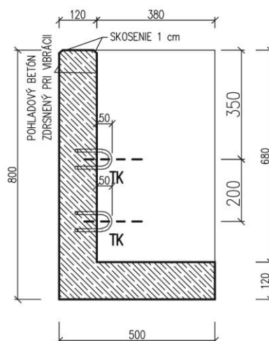
REZ A-A M=1:10
