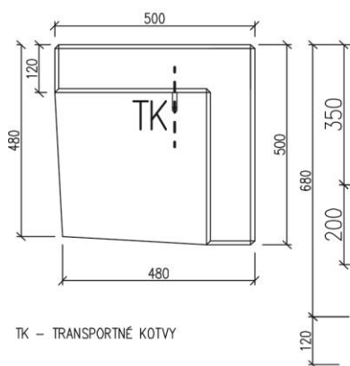
PODORYS M=1:10
