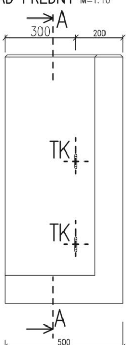
POHLAD PREDNÝ M=1:10
