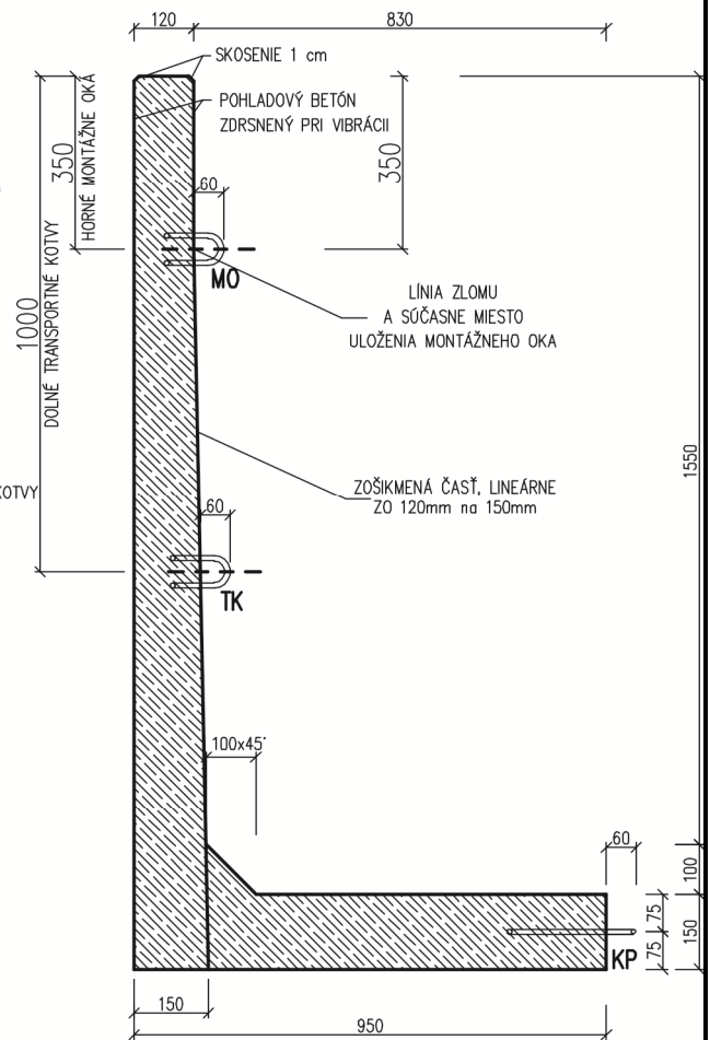
REZ A-A M=1:10
