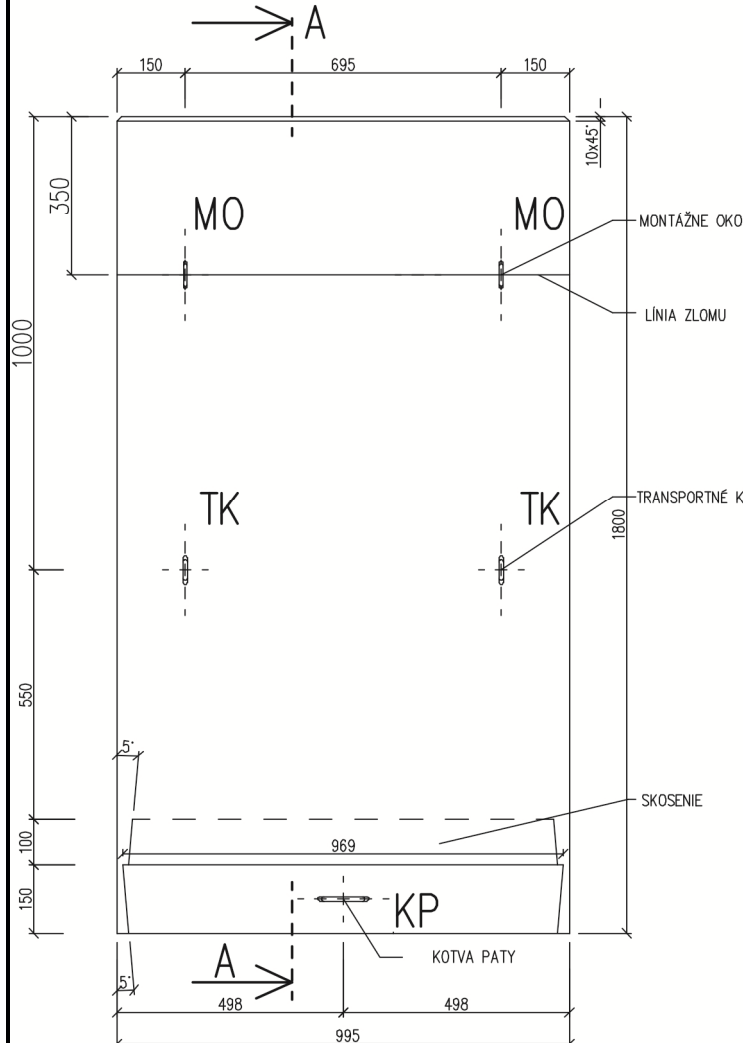
PODORYS M=1:10
