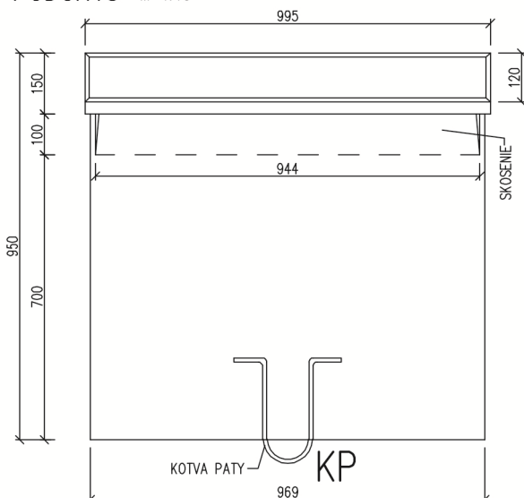
PODORYS M=1:10
