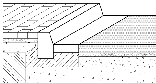
Priečne uloženie
