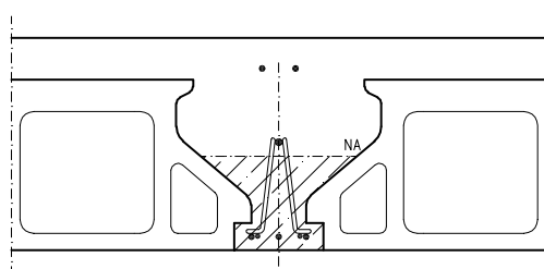
Obr. F.3 – Uvažovaný vzdorujúci prierez
