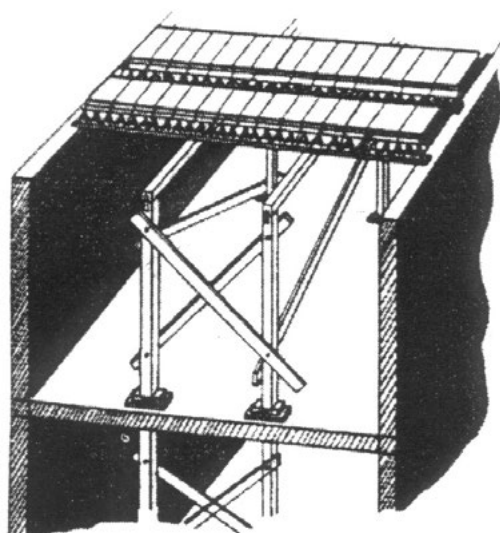
Obr. M.2 – Podperná konštrukcia
