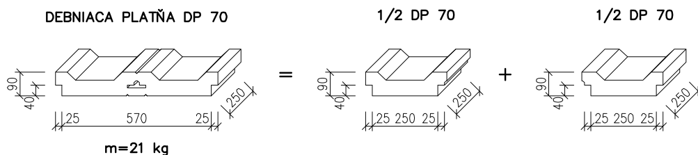
Obr. 3 – Debniaca platňa DP70
