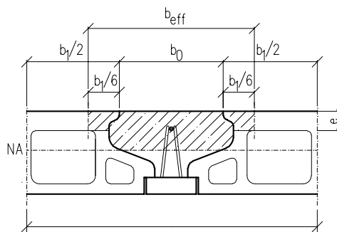
Obr. F.2 – Definícia účinnej šírky stropov 20+0 a 25+0
