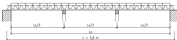
PRÍKLAD PODOPRETIA TRÁMY EN580 PRI STROPE 25+0
