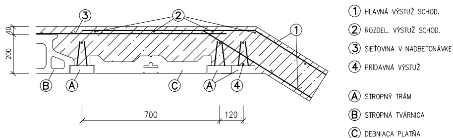
Obr. E.11 – Detail napojenia schodiska [Rez G-G]
