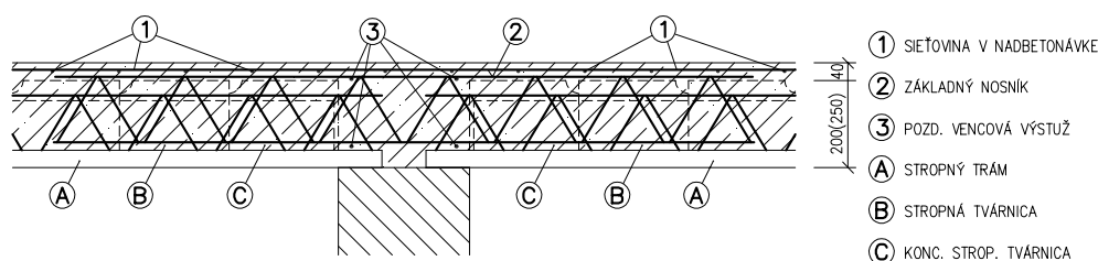
Obr. E.8 – Detail vnútornej podpery so spojitostou
