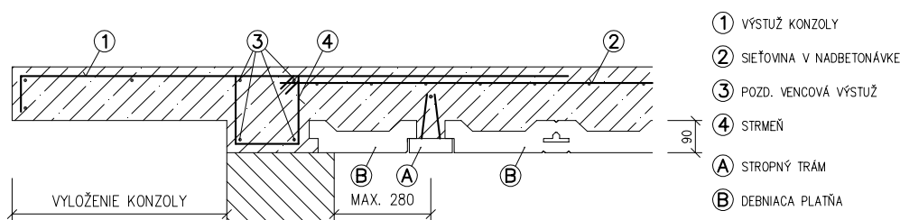
Obr. E.9 – Detail konzoly kolmo na smer trémov [Rez E-E]
