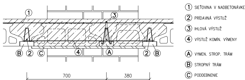
Obr. E.14 – Detail komínovej výmeny [Rez K-K]
