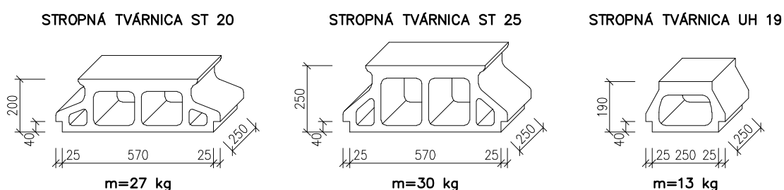
Obr. 2 – Stropná tvárnica ST20, ST25 a UH19
