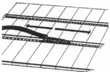
Obr. M.3 – Spôsob betónovania pomocou bádie a pumpy
