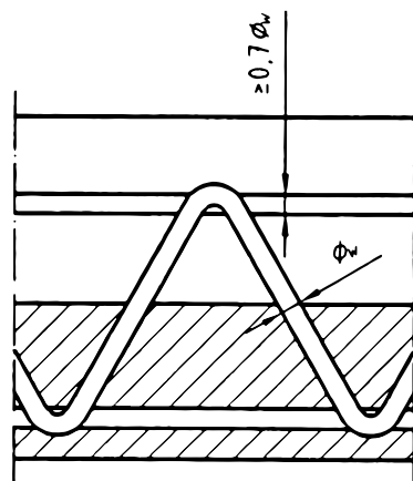
Obr. D.2 – Spojité diagonály a zvárané spoje
