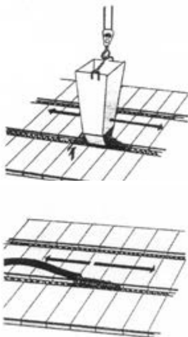
Obr. M.3 – Spôsob betónovania pomocou bádie a pumpy
