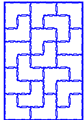
Vzor kladenia dlažby
