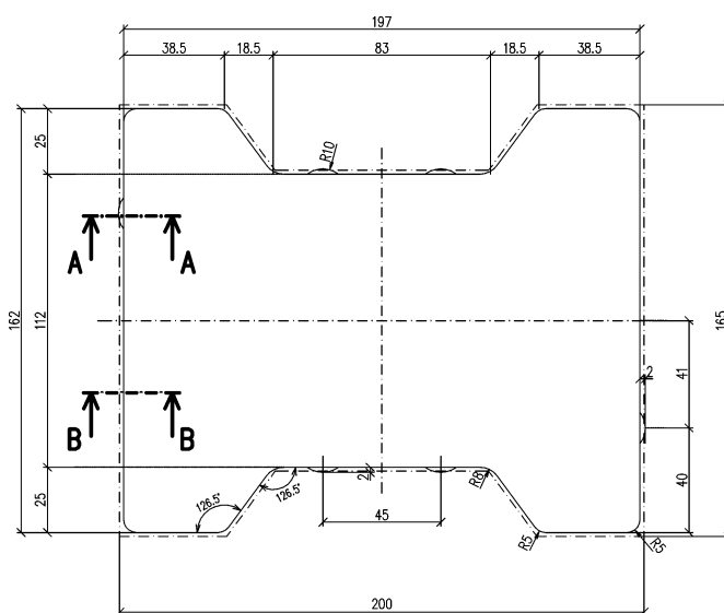
Pohl'ad zhora
