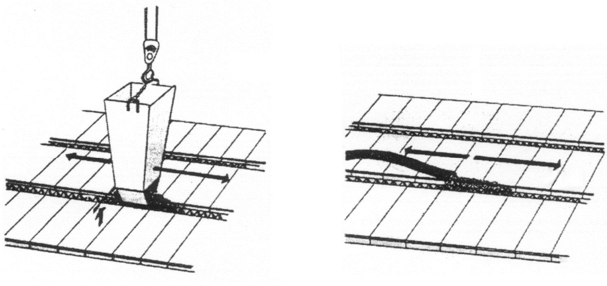
Obr. M.3 – Spôsob betónovania pomocou bádie a pumpy
