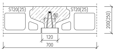
Obr. B.2 – Strop s kombinovanou nadbetónávkou
