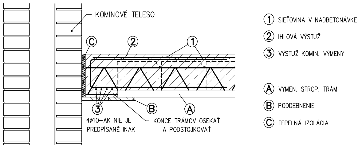
Obr. E.13 – Detail komínovej výmeny (Rez J-J)
