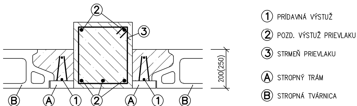
Obr. E.15 – Detail vloženého obráteného monolitického nosníka
