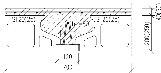
Obr. B.1 – Stropná konštrukcia so spojitou nadbetónávkou
