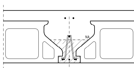
Obr. F.3 – Uvažovaný vzdurojúci prierez
