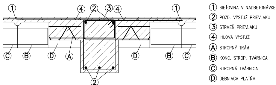
Obr. E.6 – Trámy podoprené vloženým hlavným nosníkom
