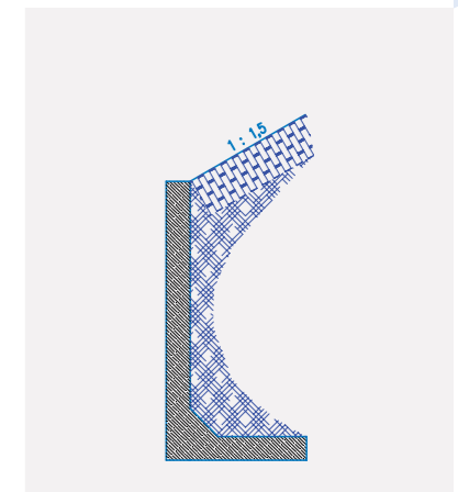
ZAŤAŽOVACÍ STAV 3A n = 1:1,5 – svah, spád terénu 33,7°
