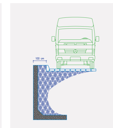
ZAŤAŽOVACÍ STAV 5 - SLW 60 premenné zaťaženie q = 33,3 \text{ kN/m}^2 diaľnica s ťažkotonnou dopravou
