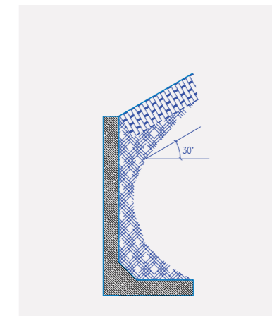
ZAŤAŽOVACÍ STAV 3 svah, spád terénu 30°
