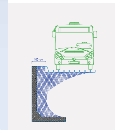
ZAŤAŽOVACÍ STAV 4 - SLW 30 premenné zaťaženie q = 16,7 \text{ kN/m}^2 verejná komunikácia s obslužnou dopravou
