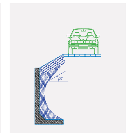
ZAŤAŽOVACÍ STAV 6 cesta na svahu, spád terénu 30°
